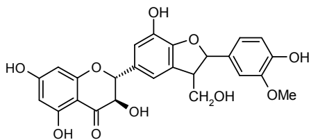
Silychristin
