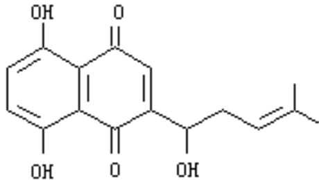
II C_{16}H_{16}O_5 MW: 288.3 CAS#: 517-89-5
