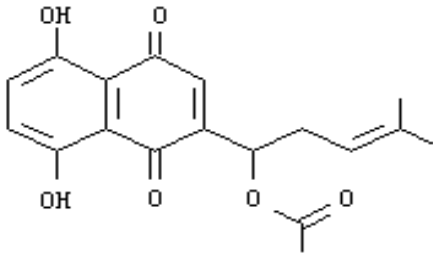
I C_{18}H_{18}O_6 MW: 330.3 CAS#: 24502-78-1
